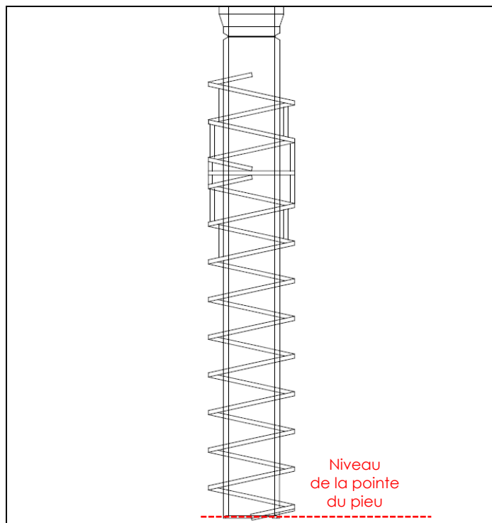
Fig. 1 : Dessin technique de la tarière prise en considération
