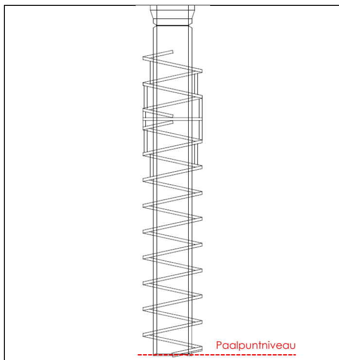
Fig. 1 : Technische schets van de beschouwde boorkop
