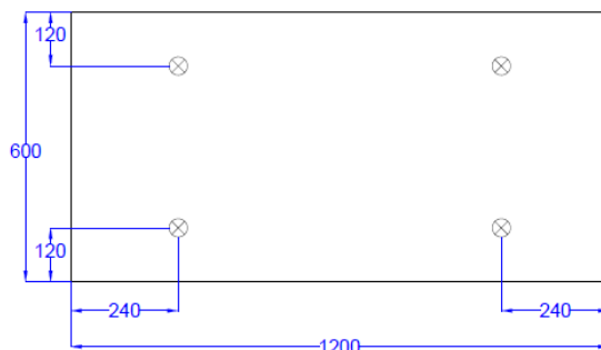
Fig. 1 – Plaatsingspatronen voor de mechanische bevestigingen
