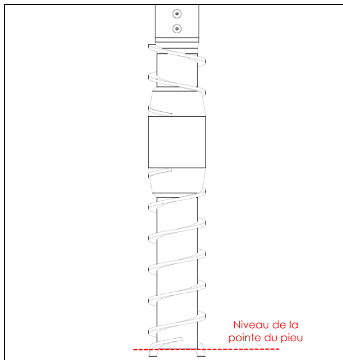
Fig. 1 : Dessin technique de la tarière
