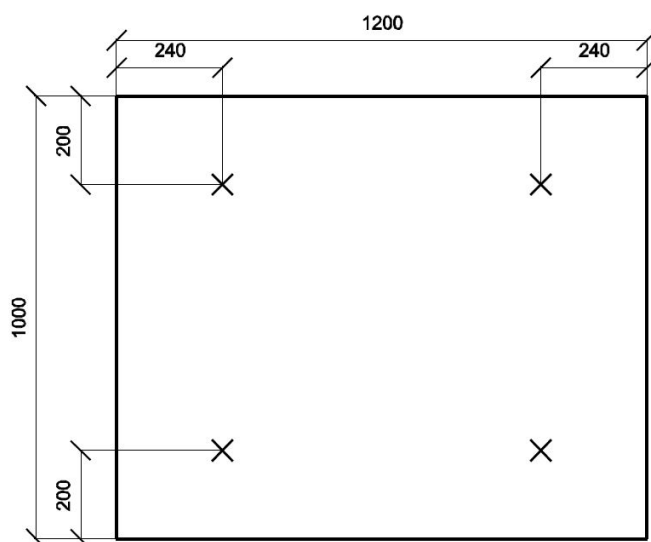
Fig. 1 – Schémas de pose pour les fixations mécaniques – dimensions en mm
