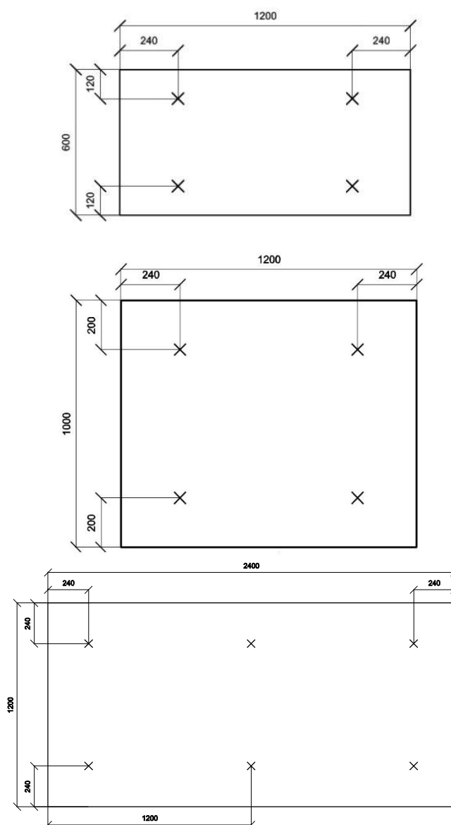
Fig. 1 – Plaatsingspatronen voor de mechanische bevestigingen – afmetingen in mm
