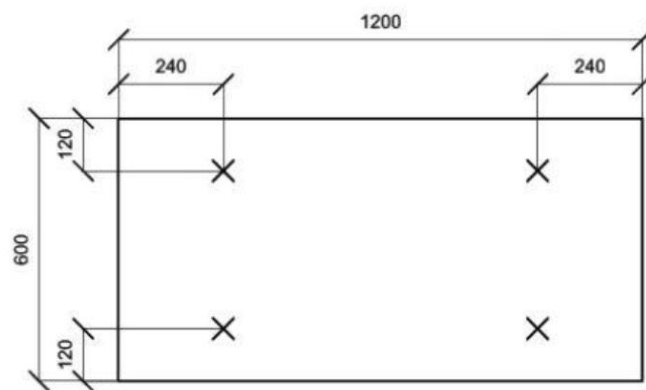
Fig. 1 Schémas de pose pour les fixations mécaniques
