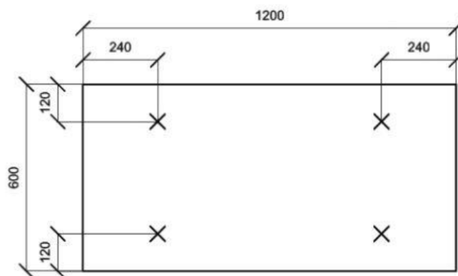
Fig. 1 Plaatsingspatronen voor de mechanische bevestigingen
