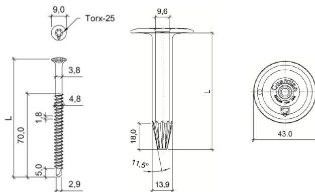
Fig. 2 – Schroef GUARDIAN BS -4.8 + telescopische tule GUARDIAN R 45
