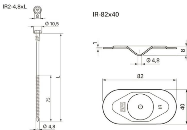
Fig. 1 – Schroef SFS IR2-4,8 + bevestigingsplaatje IR-82x40
