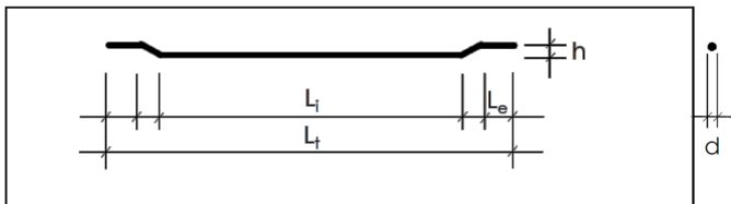
Fig. 1 – Vorm van de MPZ staalvezel
