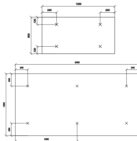
Fig. 1 – Plaatsingspatronen voor de mechanische bevestigingen – afmetingen in mm
