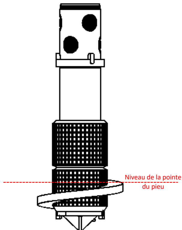
Fig. 1 : Dessin technique de la tarière
