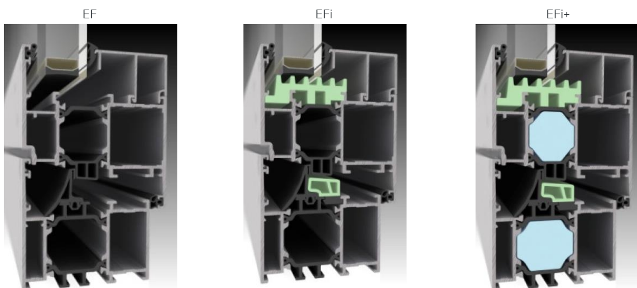
Figuur 1: Uitvoeringsvarianten
