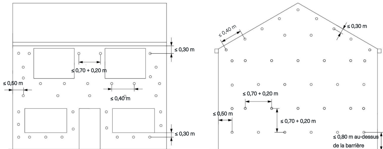
Fig. 1 Représentation schématique du schéma de remplissage dans le cas de buses d'insufflation de 14 mm
