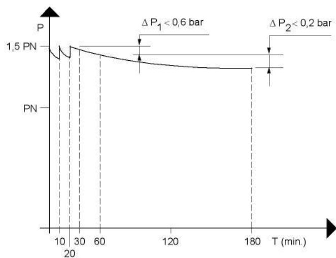
Fig. 1 : Dichtheidscontrole.
