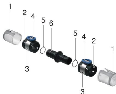
Fig. 1 voorbeeld van PPSU-koppeling
