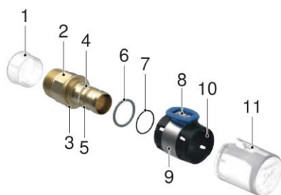
Fig. 2 voorbeeld van metalen koppeling
