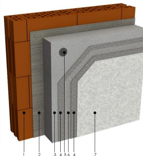
Fig. 1 – Opbouw van het ETICS (External Thermal Insulation Composite Systems)
