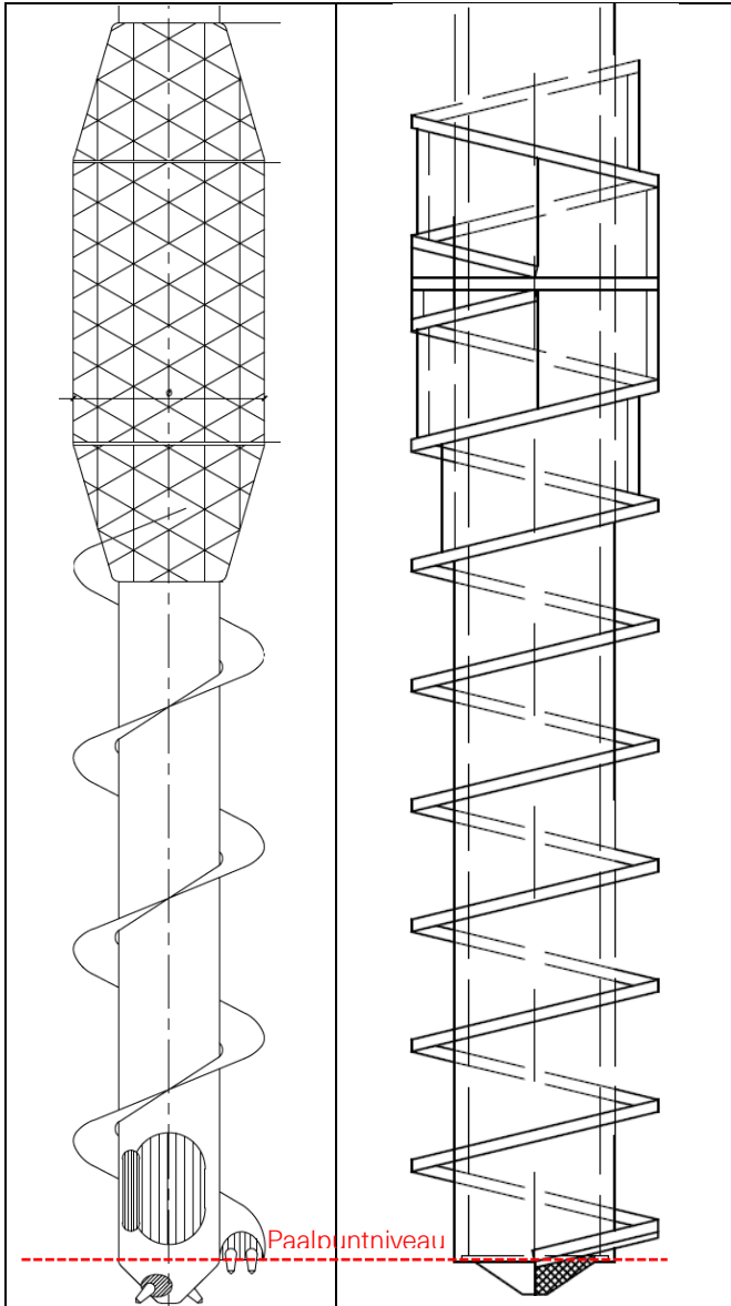
Figuur 1: Technische schets van de beschouwde boorkop
