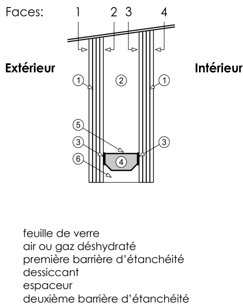
Figure 1 – Faces d'un vitrage isolant
