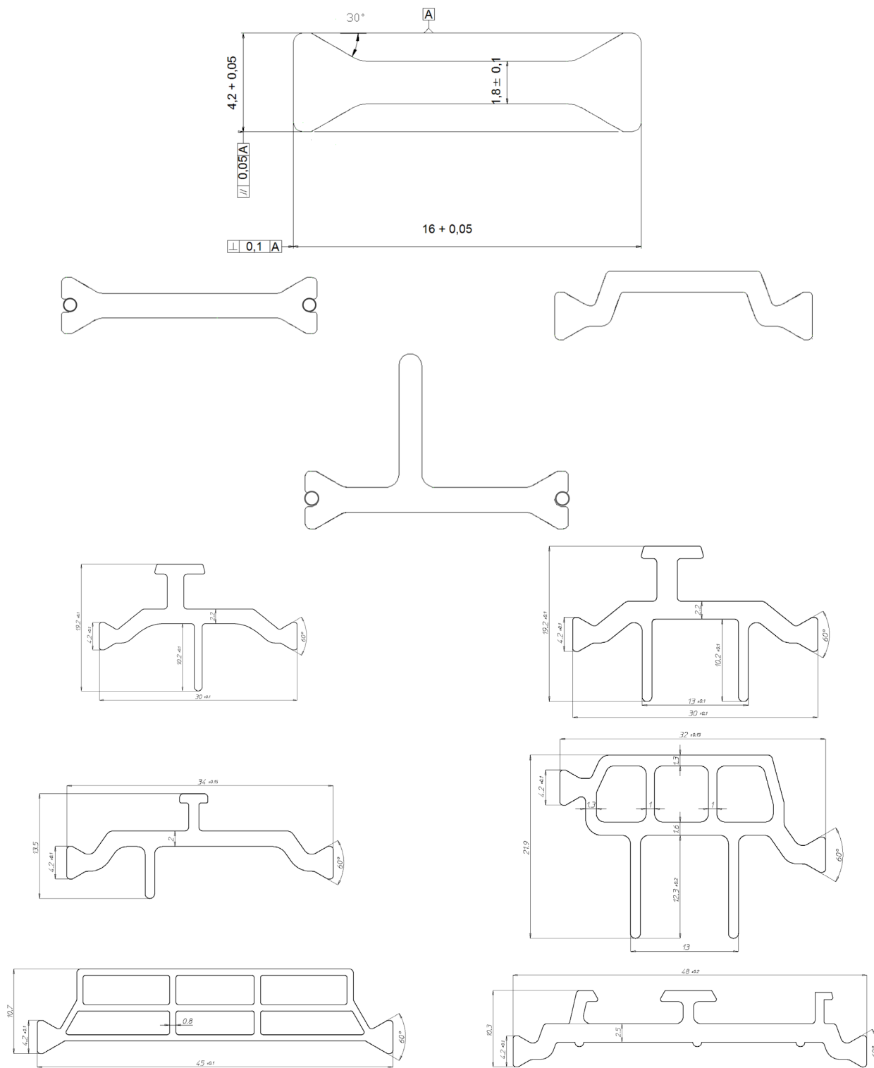
Figuur 2 : Voorbeeld plaatsing strippen
