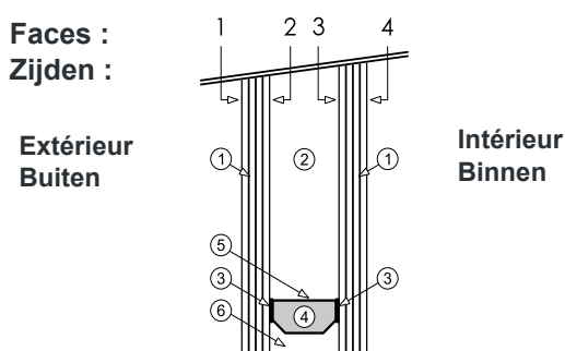
Fig. 1 – Faces d'un vitrage isolant
