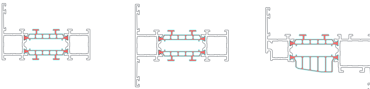
Fig. 4: Système Star
