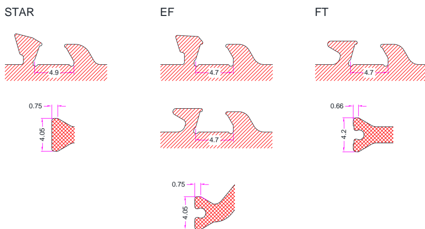
Fig. 2: Système Futural
