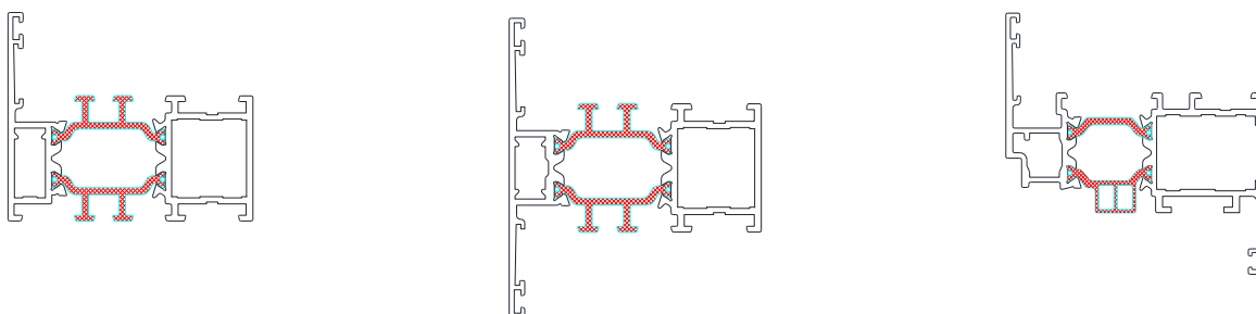
Fig. 4: Système Star
