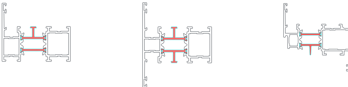
Fig. 3: Système EcoFutural
