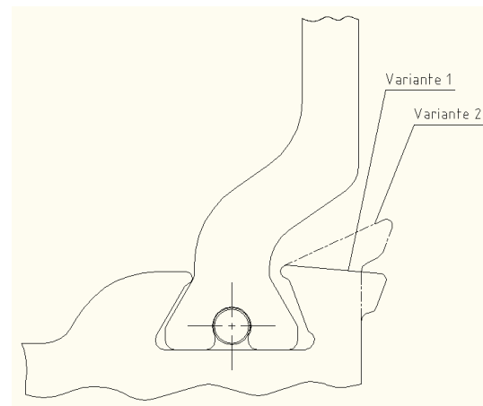
Figure 2 : Exemple de pose de barrettes
