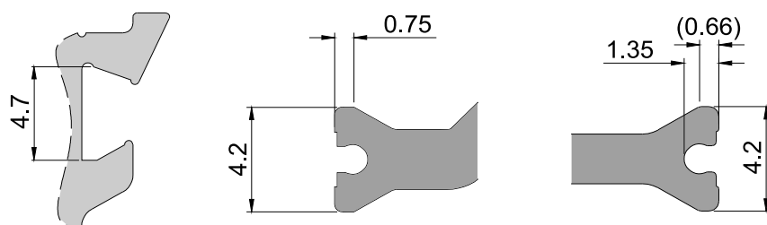
Figure 1 - Géométrie des pattes de serrissage et du talon de barrette
