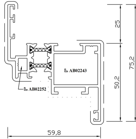
profilé RP 1702T
