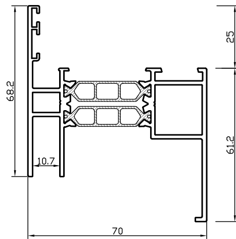
profilé RP 1882T
