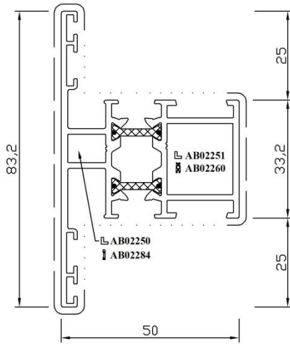
profilé RP 1703T
