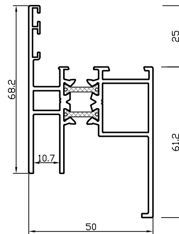
profilé RP 1782T
