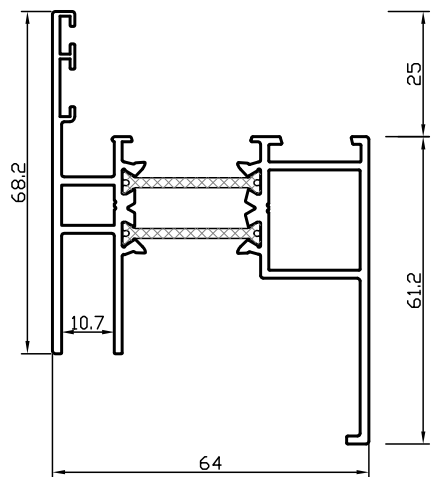
profilé RP 1282T
