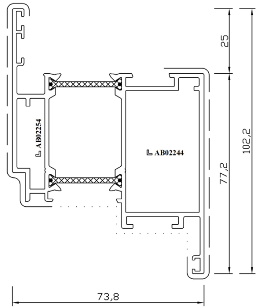
profilé RP 1204T
