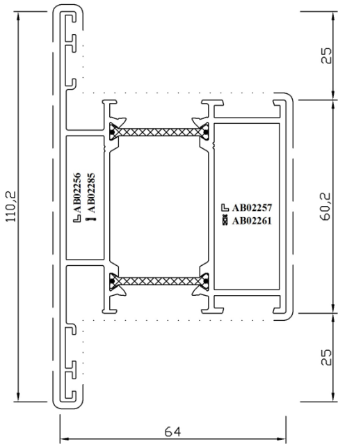
profilé RP 1205T
