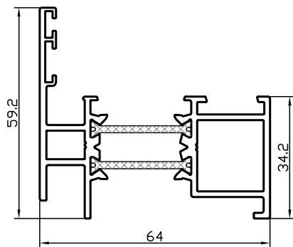
profilé RP 1281T
