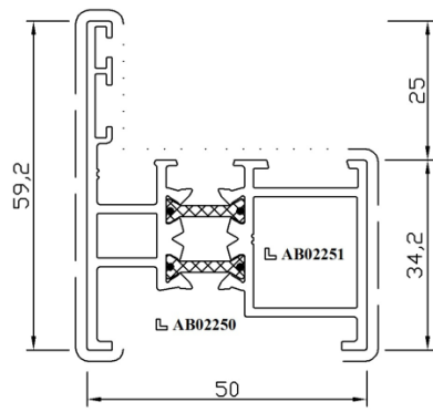
profilé RP 1701T
