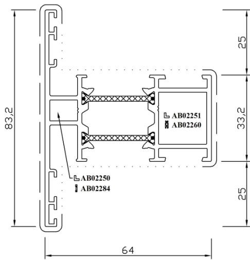
profilé RP 1203T
