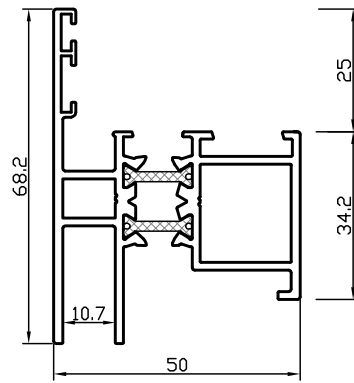
profilé RP 1772T
