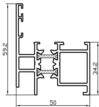
profilé RP 1781T
