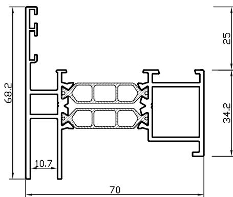
profilé RP 1881T
