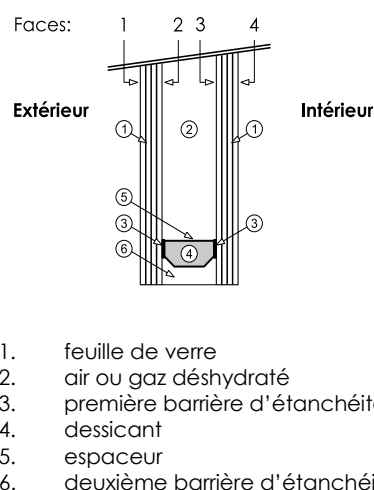
Fig. 1 – Faces d'un vitrage isolant
