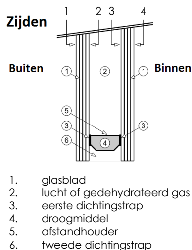
Fig. 1 – Zijden van een isolerende beglazing
