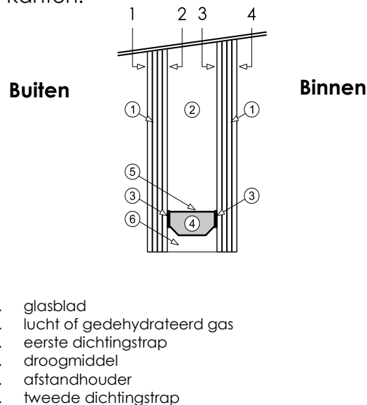
Figuur 1 – Kanten van een isolerende beglazing
