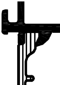
Fig. 2 – Exemple de pose de barrettes
