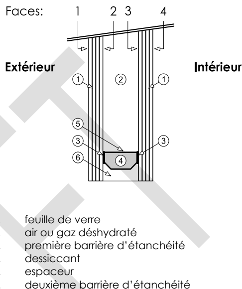
Figure 1 – Faces d'un vitrage isolant
