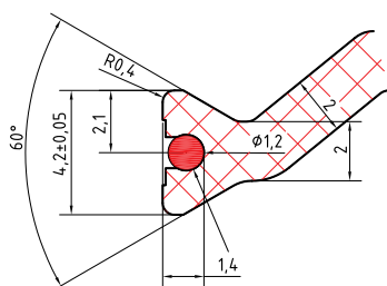
Figure 2 : Talon de barrette PA
