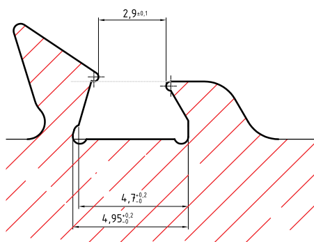
Figure 2 : Talon de barrette PET
