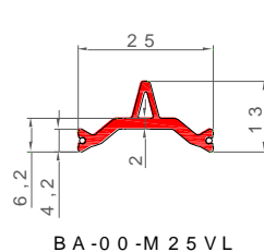
Figure 5 : Coupures thermiques – système d'assemblage Triton (barrettes PA)
