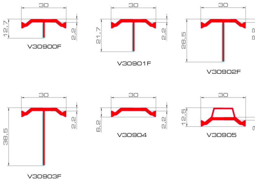
Figure 7: Coupures thermiques – systèmes d'assemblage Ventá (barrettes ABS)
