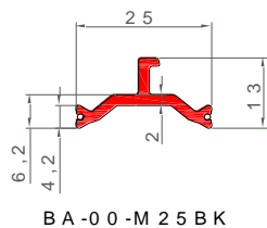
Figure 5 : Coupures thermiques – système d'assemblage Triton (barrettes PA)
