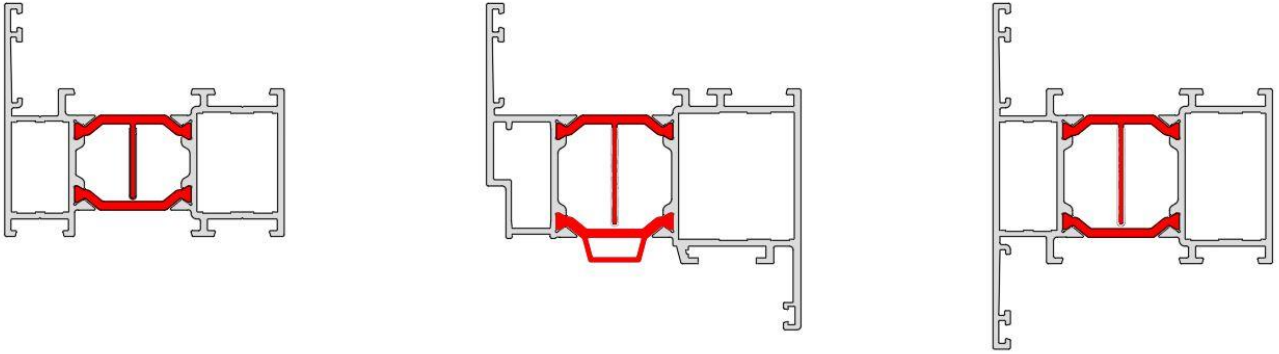
Figure 10 : Système Ventá
