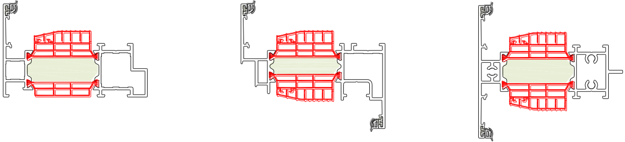
Figure 10 : Système Ventá
