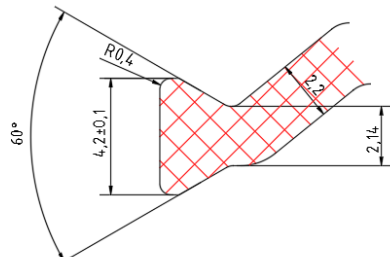
Figure 5 : Coupures thermiques – système d'assemblage Triton (barrettes PA)
