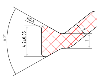
Figure 5 : Coupures thermiques – système d'assemblage Triton (barrettes PA)
