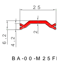
Figure 5 : Coupures thermiques – système d'assemblage Triton (barrettes PA)
