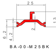
Figure 5 : Coupures thermiques – système d'assemblage Triton (barrettes PA66GF25)
