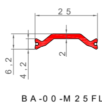
Figure 5 : Coupures thermiques – système d'assemblage Triton (barrettes PA66GF25)
