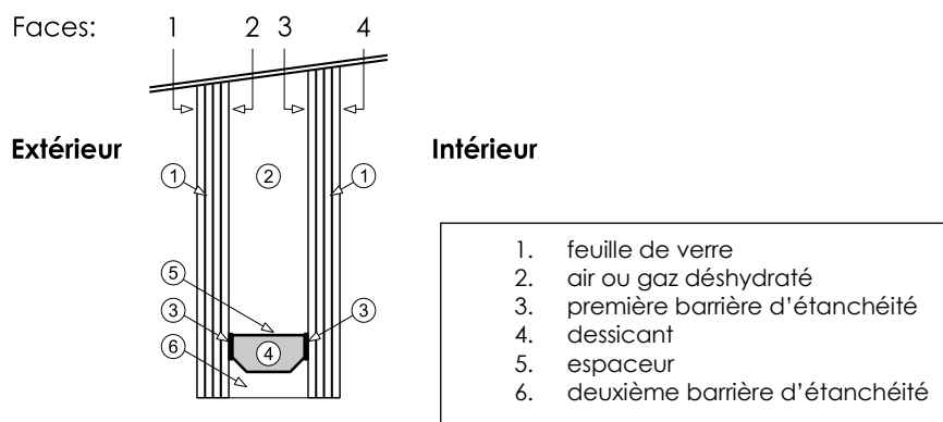
Fig. 1: Faces d'un un vitrage isolant
