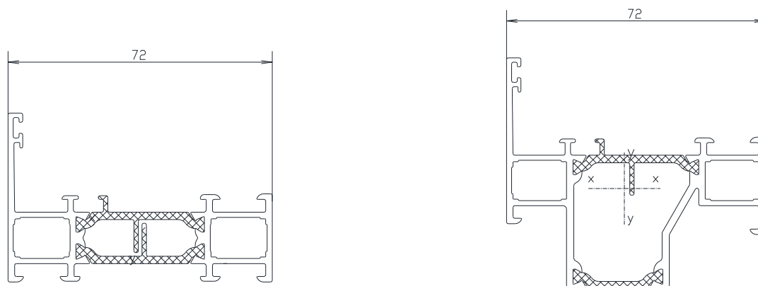
Figuur 6: Systeem RT 72, RT 72 REFLEX EN RT 72 HI+
