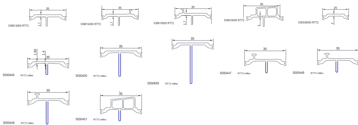
Figuur 4: Thermische onderbrekingen in PA66GF25
