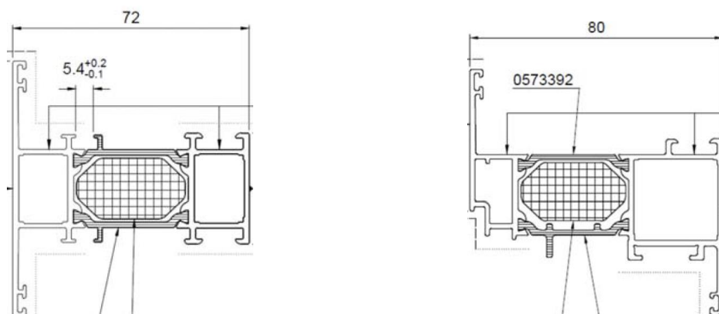
Figuur 8: Systeem RT 72 HI+
