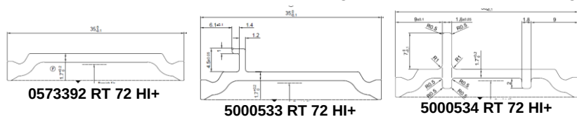
Figuur 5: Thermische onderbrekingen in ABS
