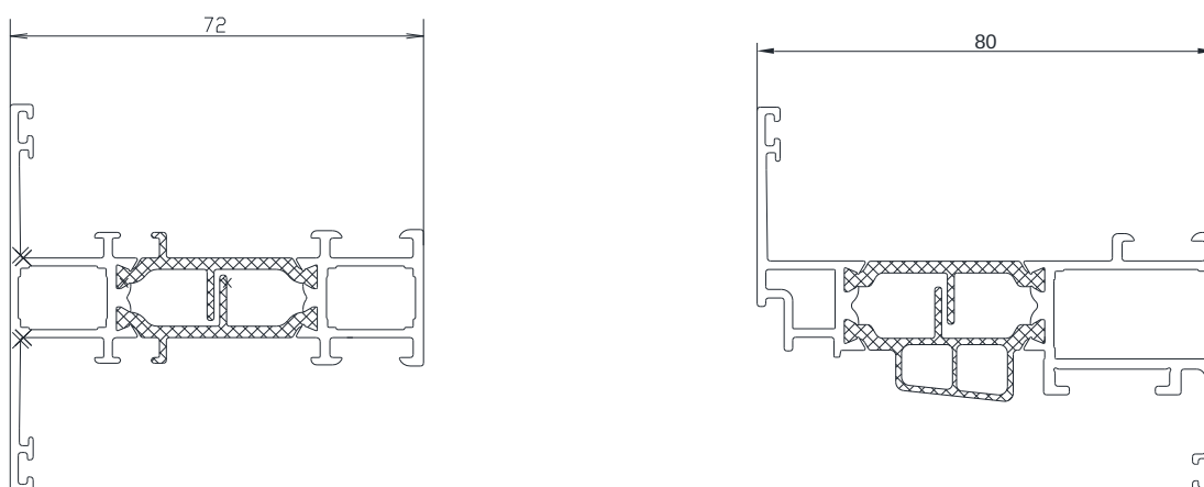
Figuur 7: Systeem RT 72 REFLEX
