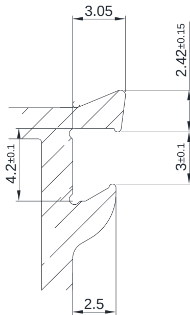
Figuur 1: Inklemmingstanden verbindingssysteem RT 72, RT 72 REFLEX en RT 72 HI+
