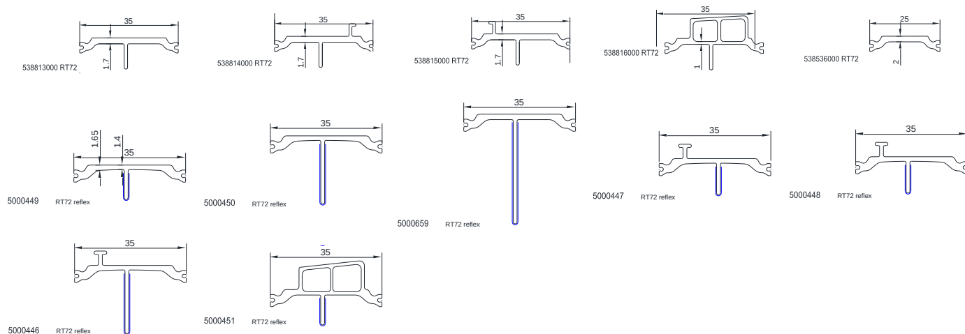
Figuur 3: Thermische onderbrekingen – verbindingssysteem (PA strippen)
