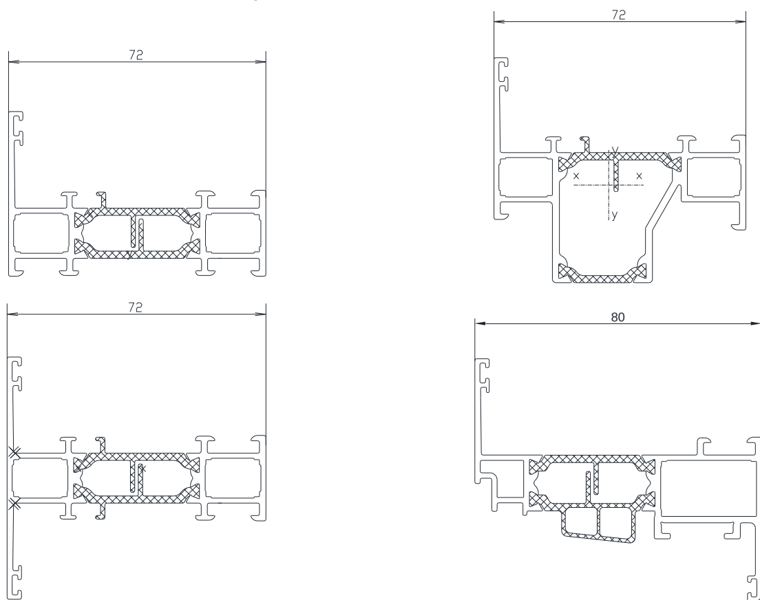
Figuur 4: Systeem RT 72 EN RT 72 REFLEX
