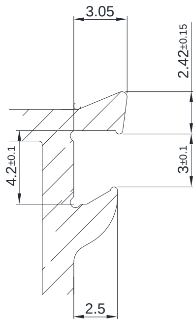
Figuur 2: PA Stripvoet
