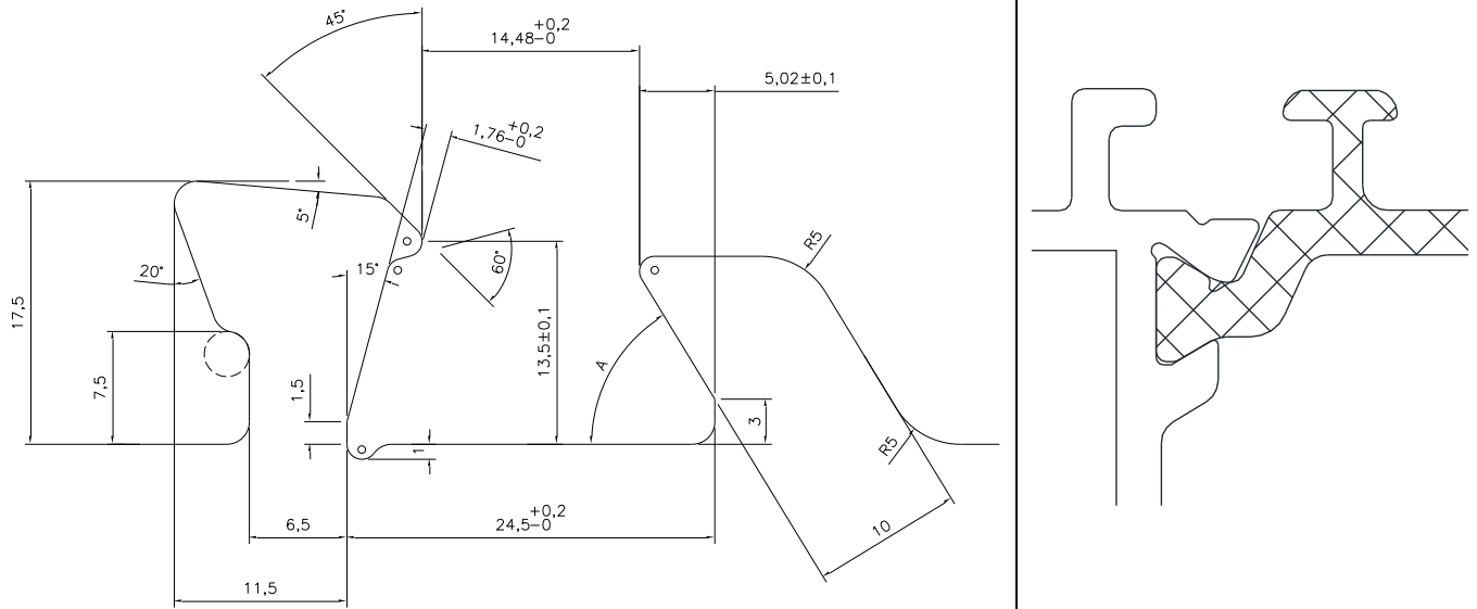
Figure 1 – Géométrie des pattes de sertissage et du talon de barrette
