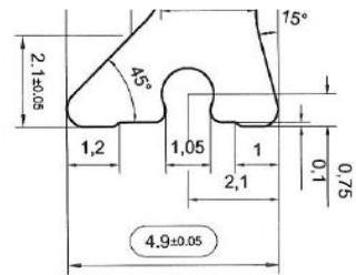
Figure 1 – Géométrie des pattes de sertissage et du talon de barrette
