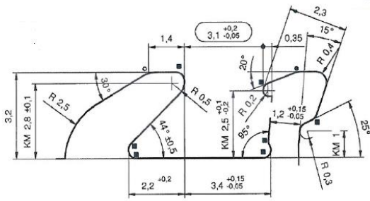
Figure 1 – Géométrie des pattes de sertissage et du talon de barrette
