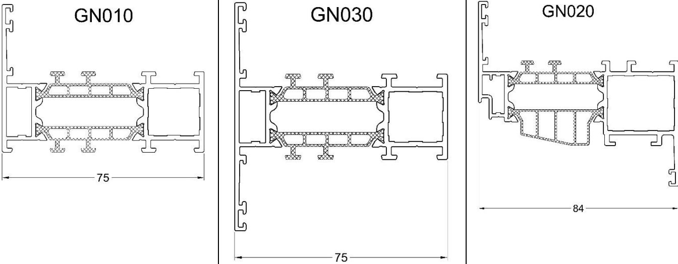
Figure 3 – Exemple Aliplast Genesis 75 fenêtres
