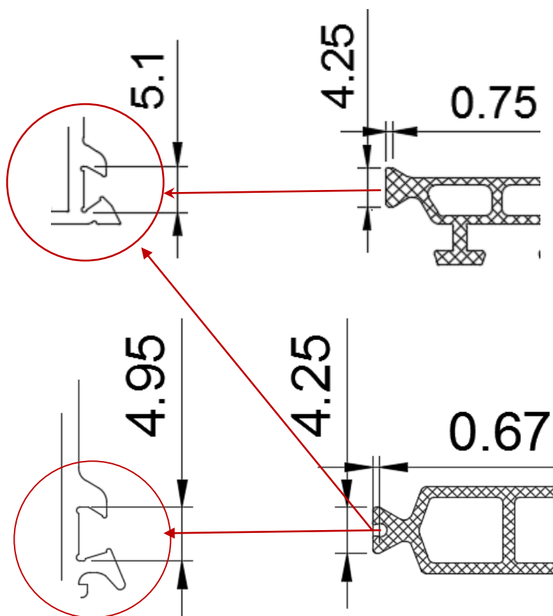
Figure 1 – Géométrie des pattes de sertissage et du talon de barrette
