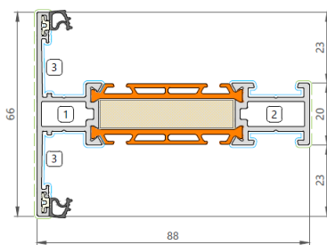
Figuur 4: Decalu 88 standaard systeem
