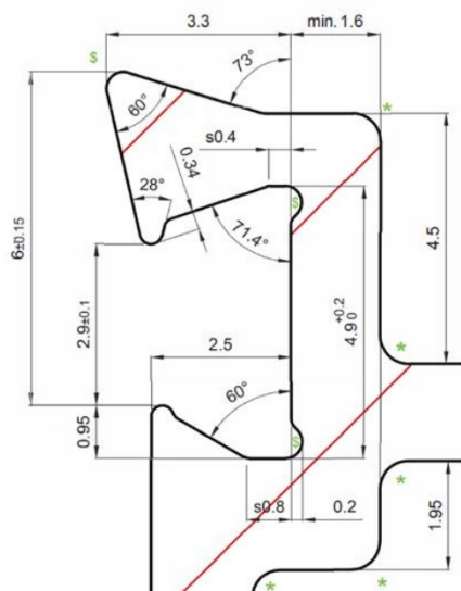
Figuur 1: Inklemmingstanden verbindingssysteem Decalu 88 standaard
