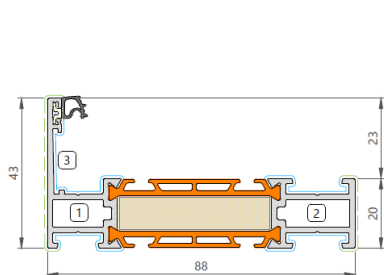
Figuur 3: Thermische onderbrekingen – verbindingssysteem Decalu 88 standaard (ABS strippen)
